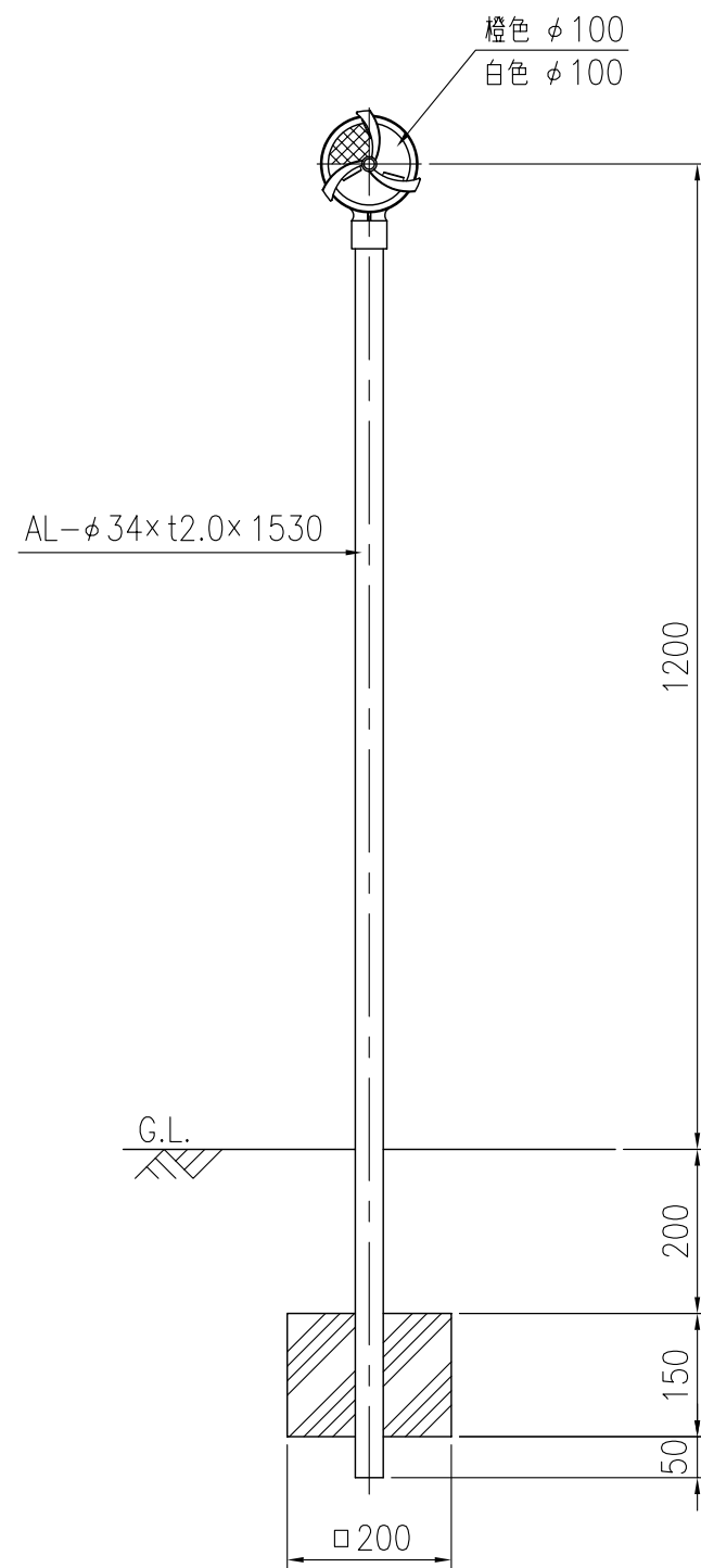
設置図 S=1/10
