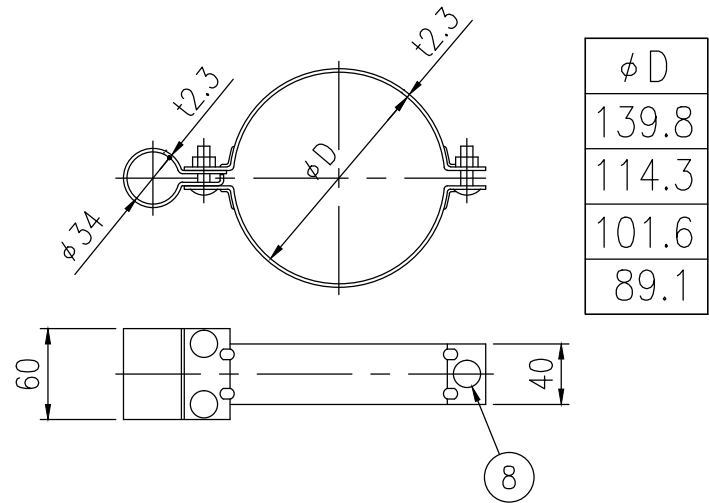
⑦ 親子バンド詳細図 S=1/5
