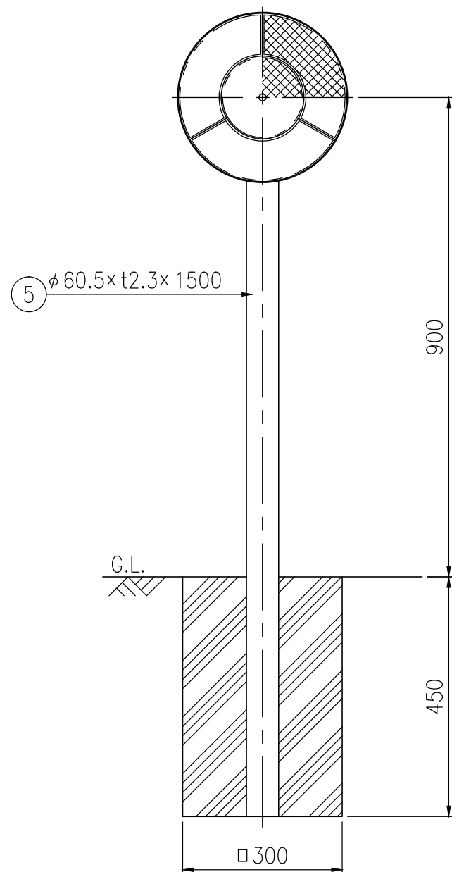
設置図 S=1/10
