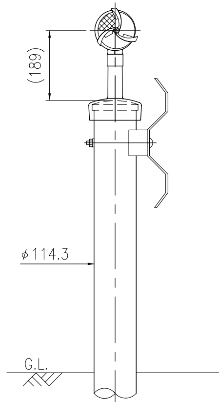
設置図 S=1/10
