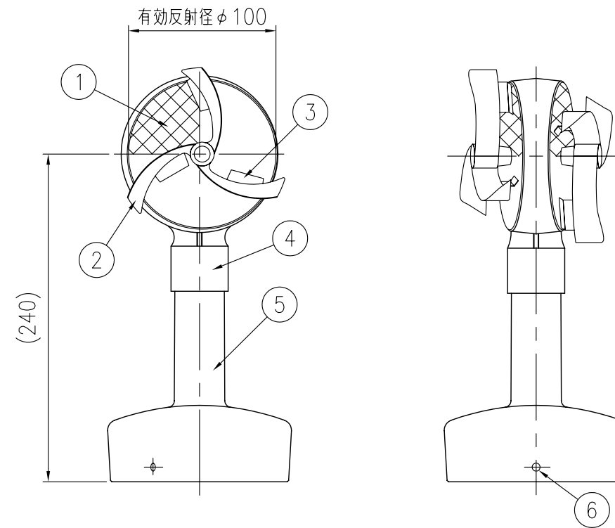
反射部詳細図 S=1/4
