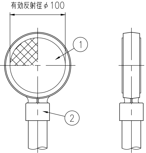
反射部詳細図 S=1/4
