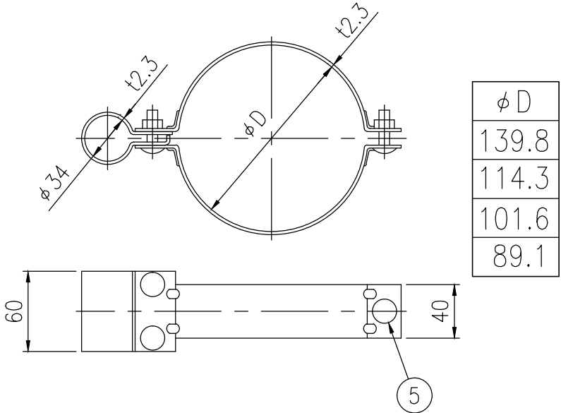
④ 親子バンド詳細図 S=1/4
