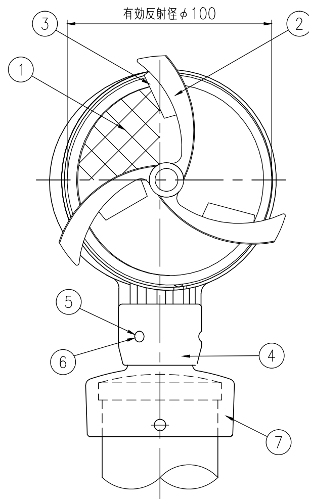
反射部詳細図 S=1/4
