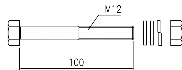
④ 金具取付ボルト S=1/2
