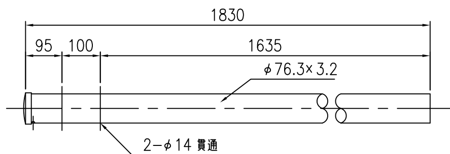
⑥ 支柱 S=1/10
