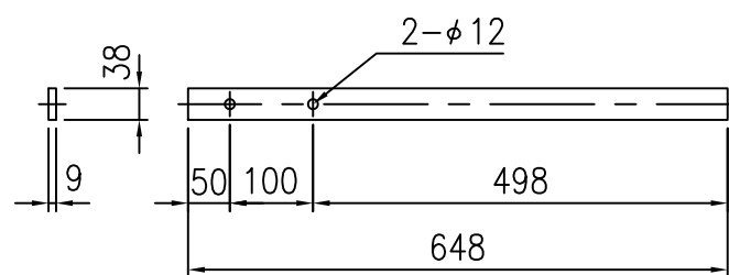
② 支脚 S=1/10
