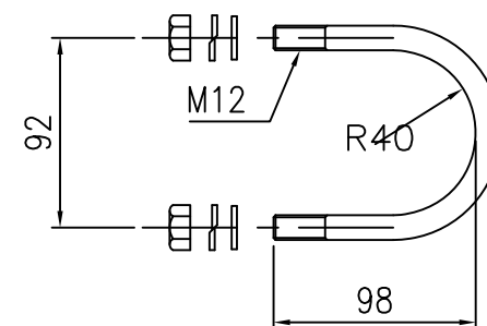
⑧ Uボルト S=1/4
