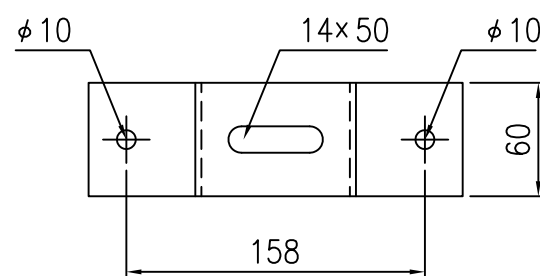
③ 取付金具 S=1/4
