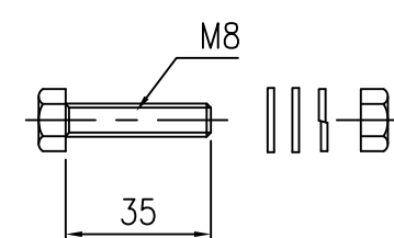
⑤ 脚取付ボルト S=1/2
