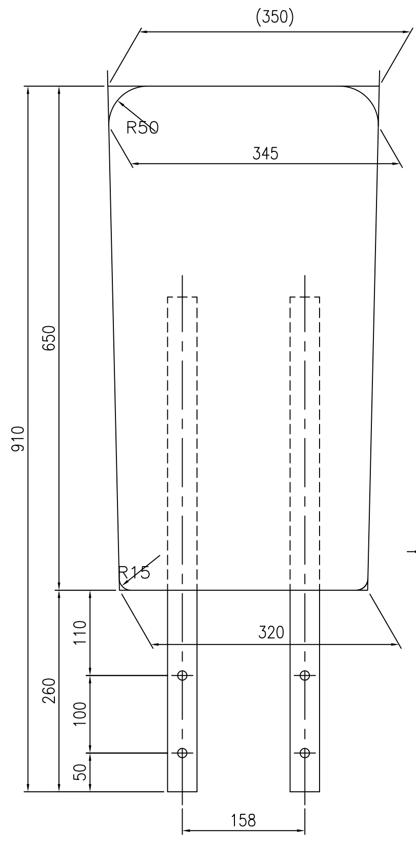
① 防眩板 S=1/5
