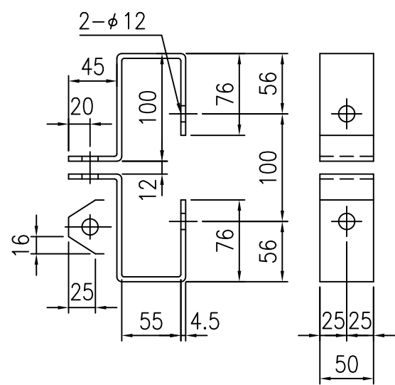
③ 取付金具 S=1/5
