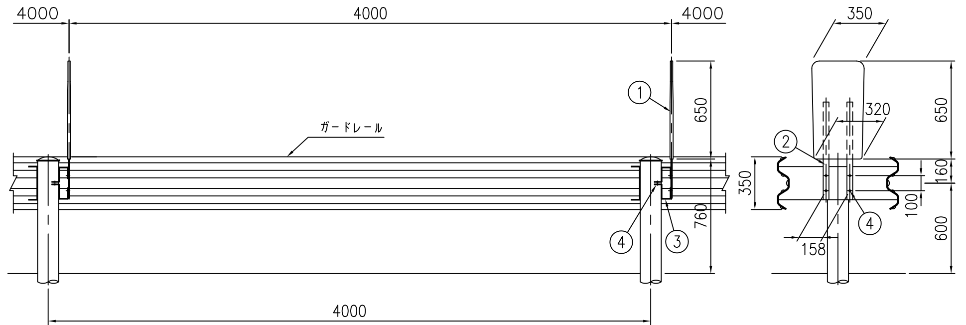
設置図 S=1/25
