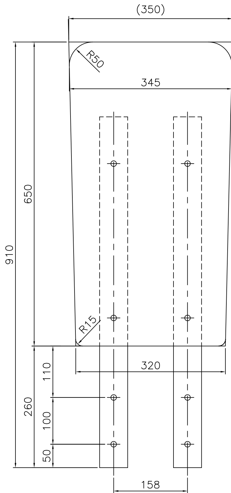
①防眩板 S=1/5
