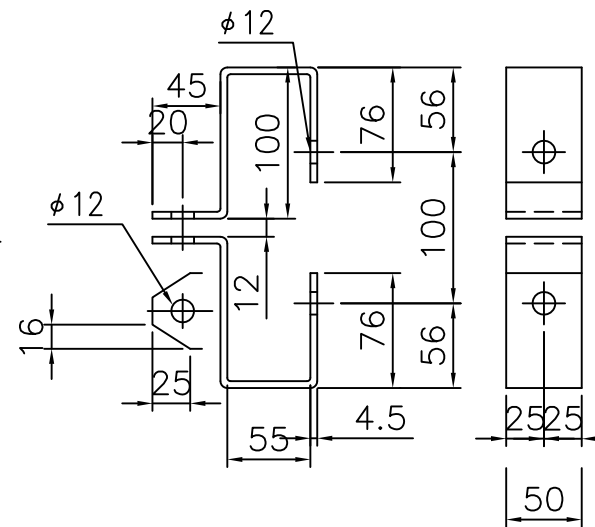
③取付金具 S=1/5
