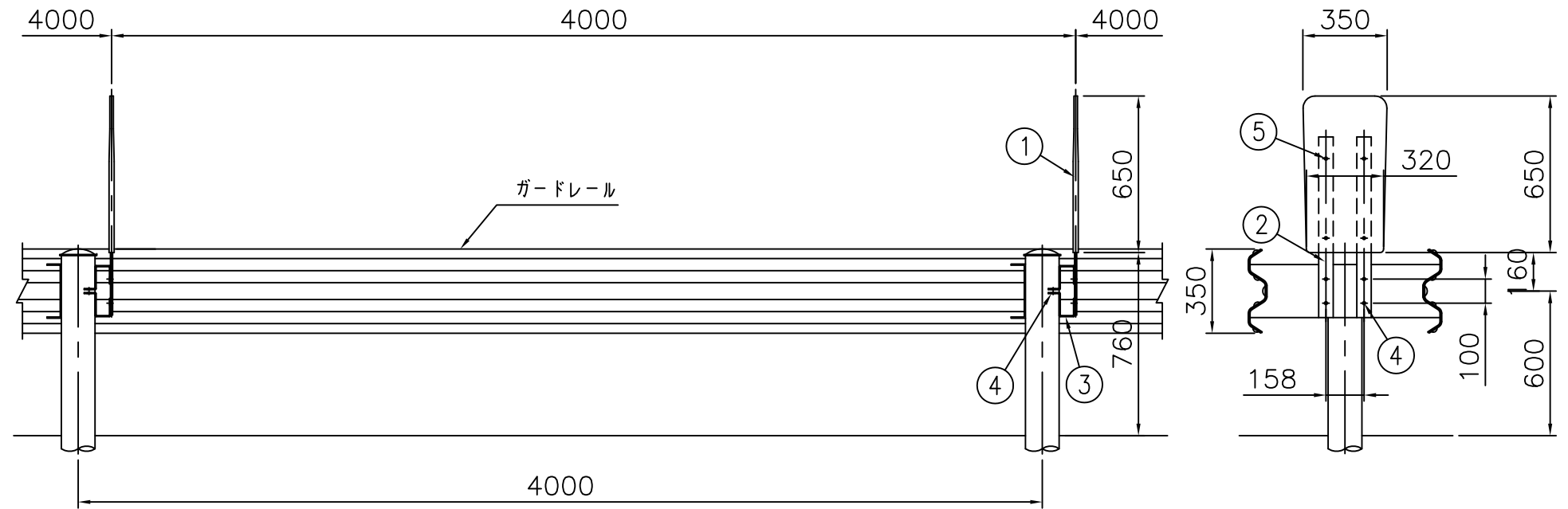
設置図 S=1/25
