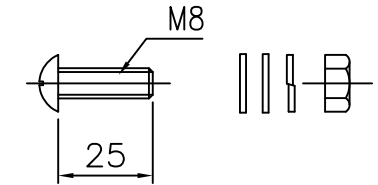
⑤防眩板取付ボルト S=1/2
