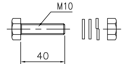
⑤防眩板取付ボルト S=1/2
