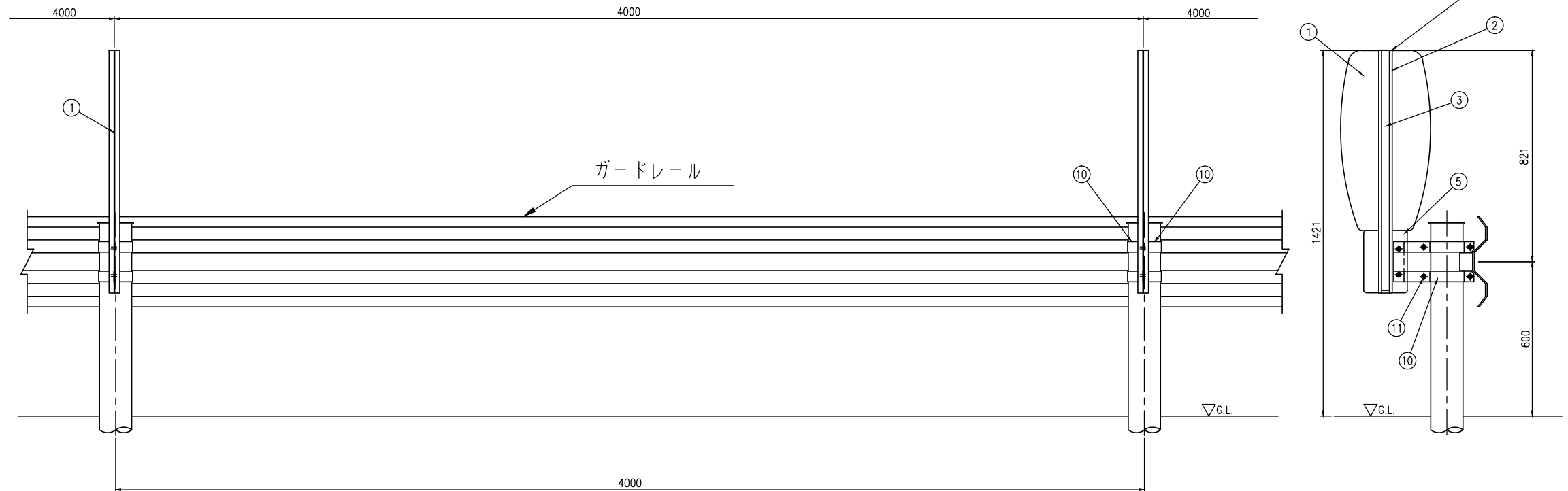
設置図 (S=1/10)
