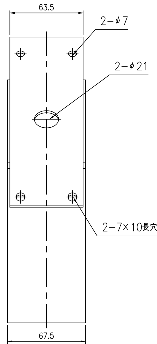
正面図
