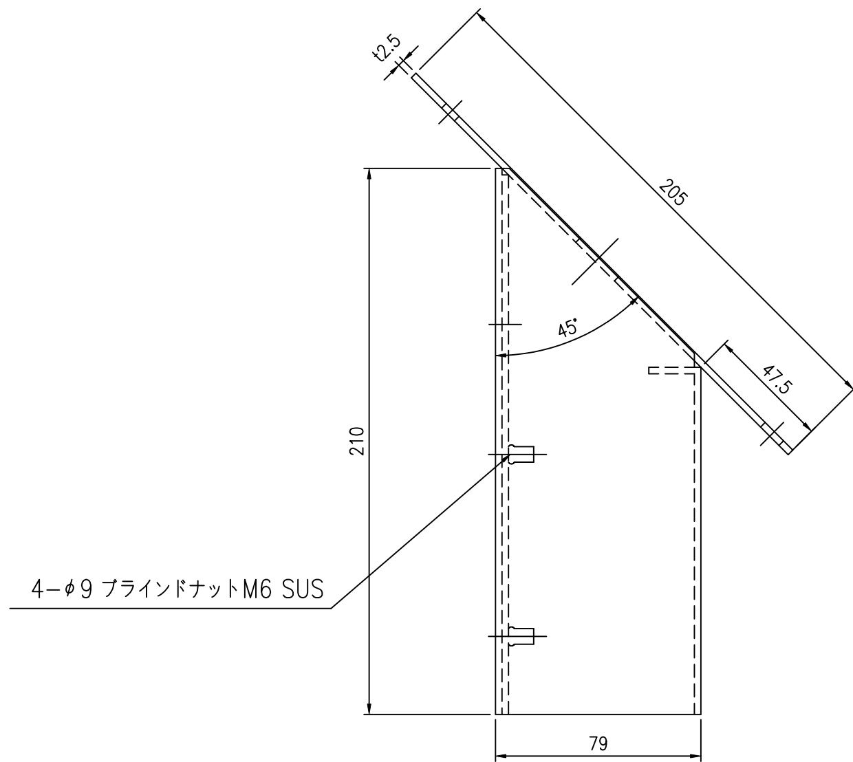
側面図
