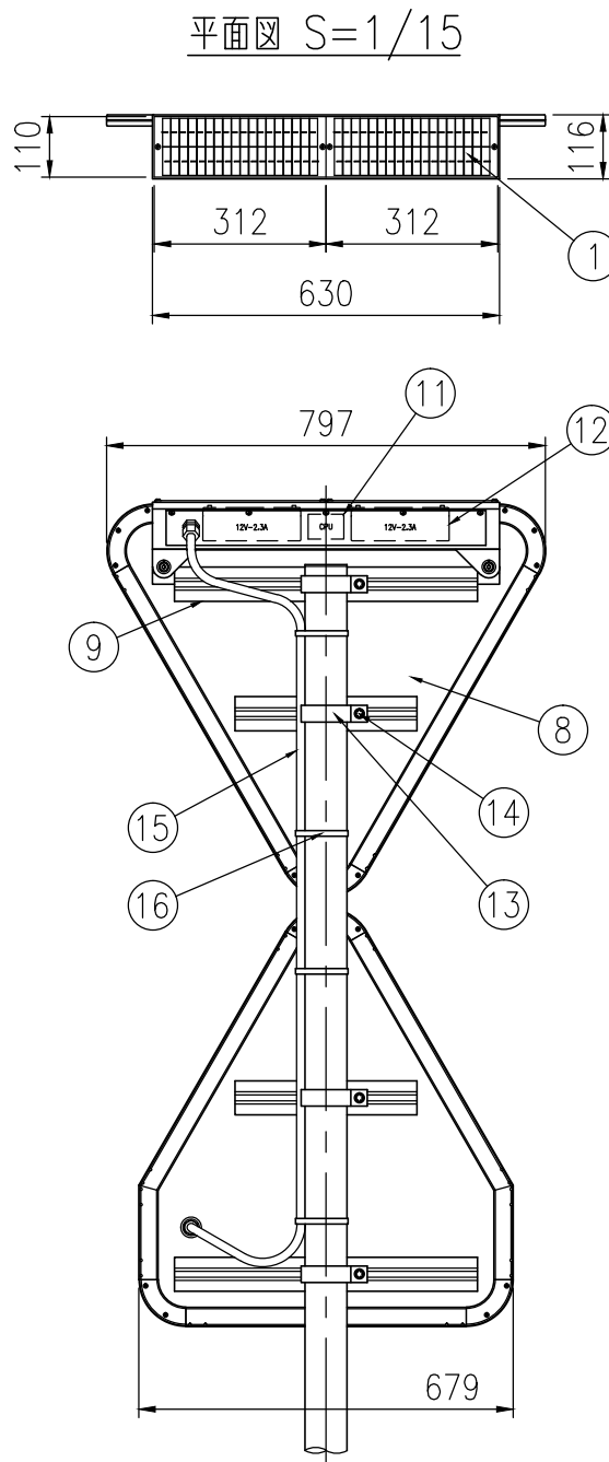
背面図 S=1/15
