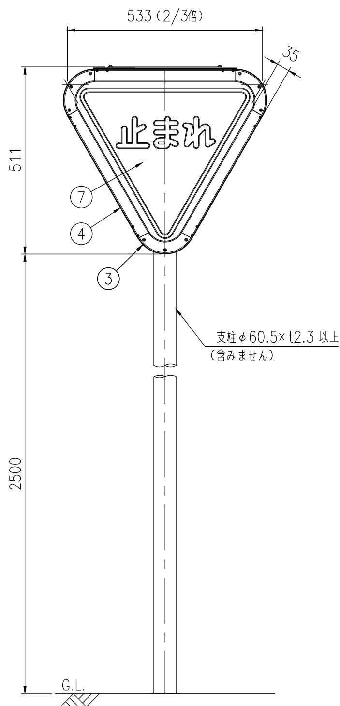
正面図 S=1/10
