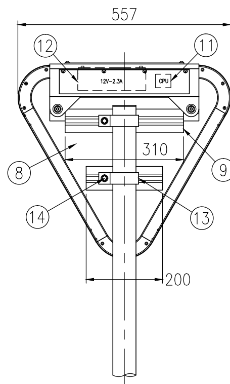
背面図 S=1/10
