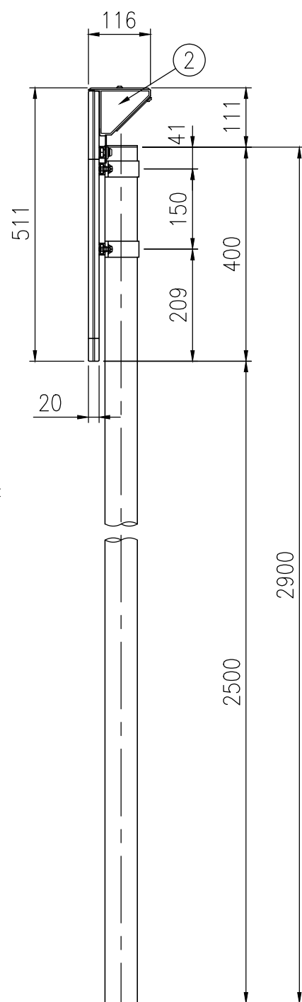
側面図 S=1/10
