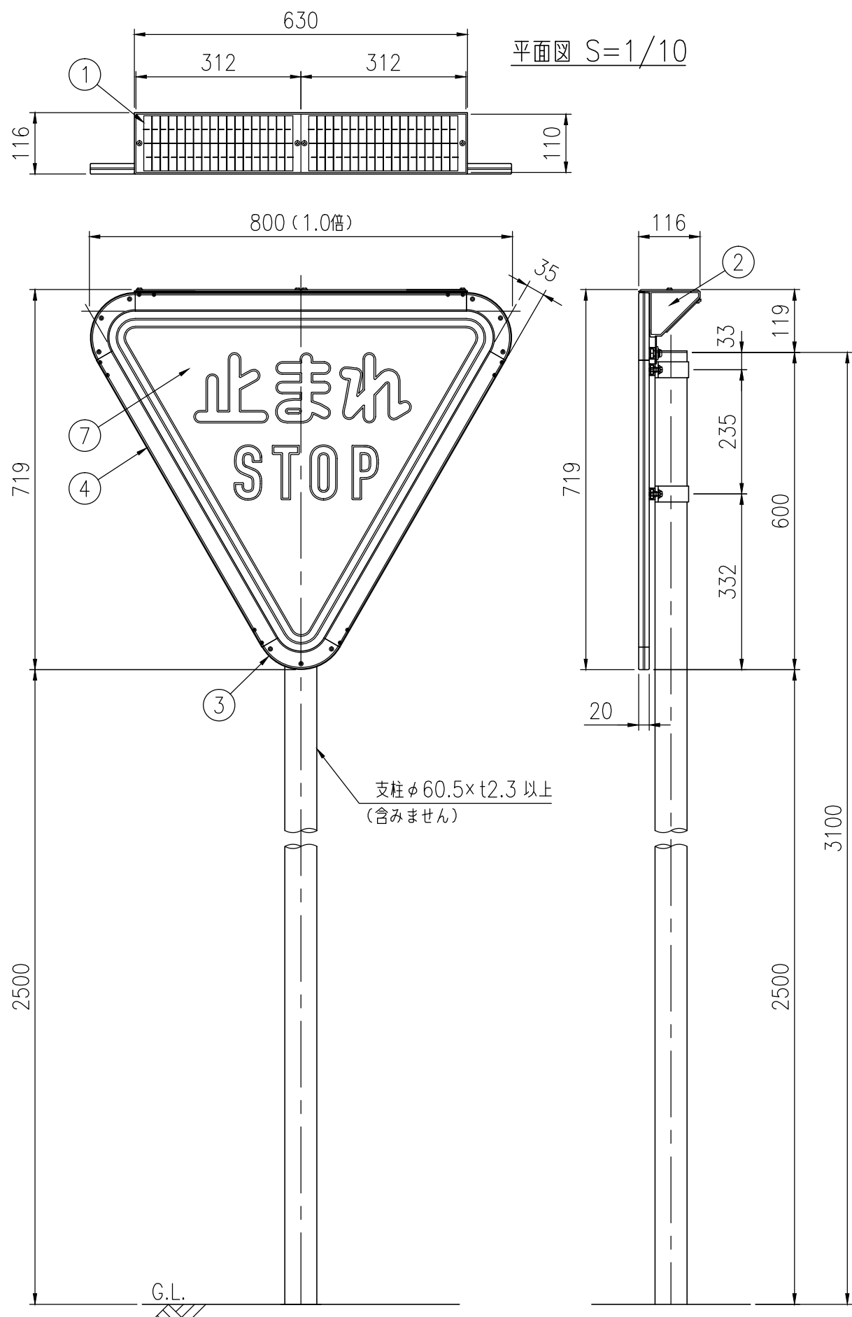
正面図 S=1/10
