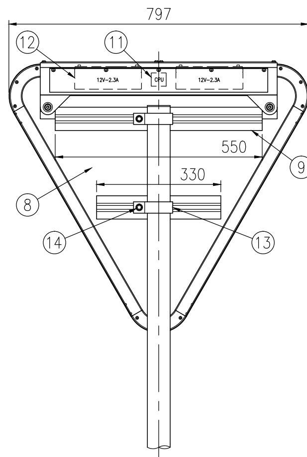
背面図 S=1/10
