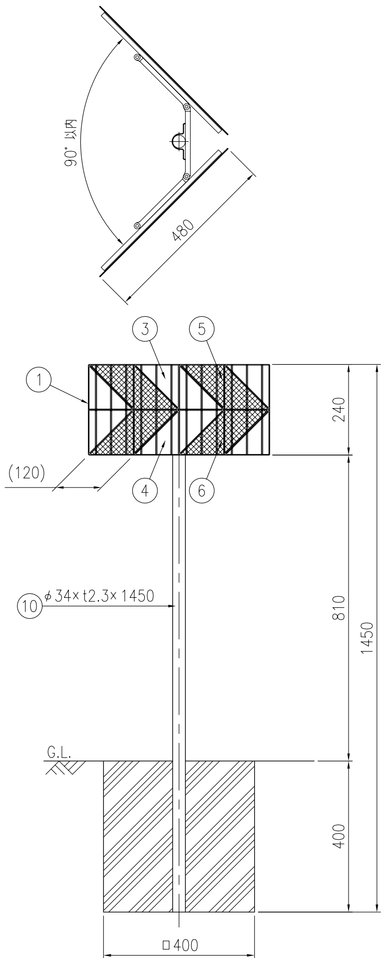
設置図 S=1/10
