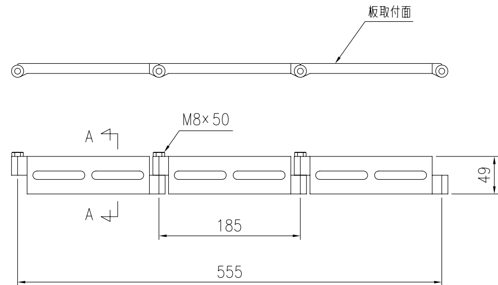
⑫ W取付金具詳細図 S=1/5
