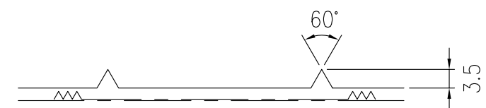
裏面図 S=1/5
