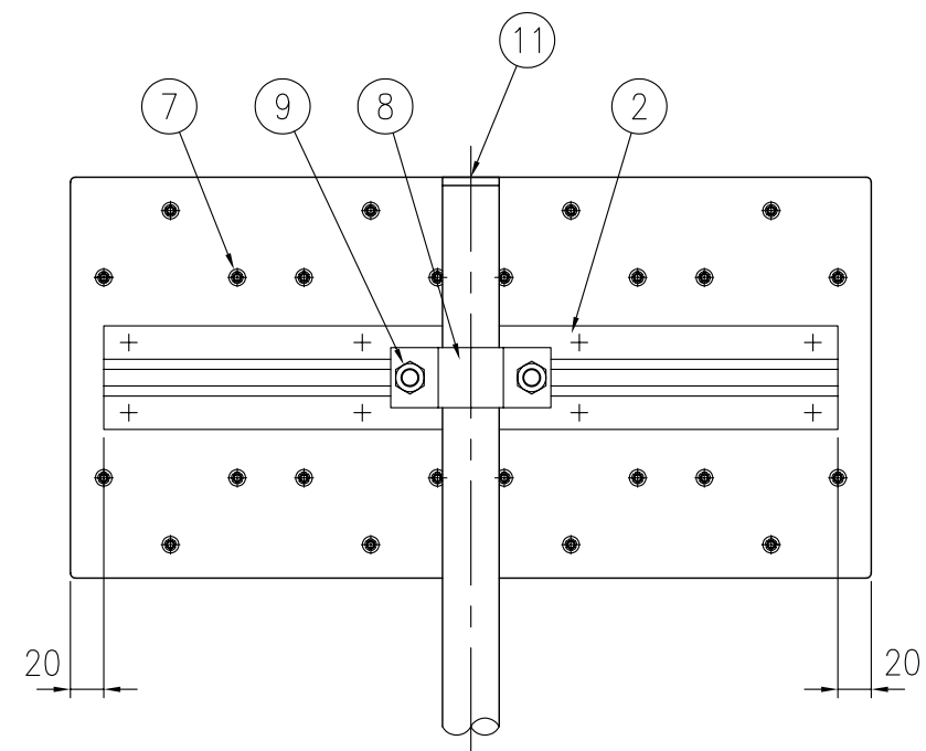
裏面図 S=1/5
