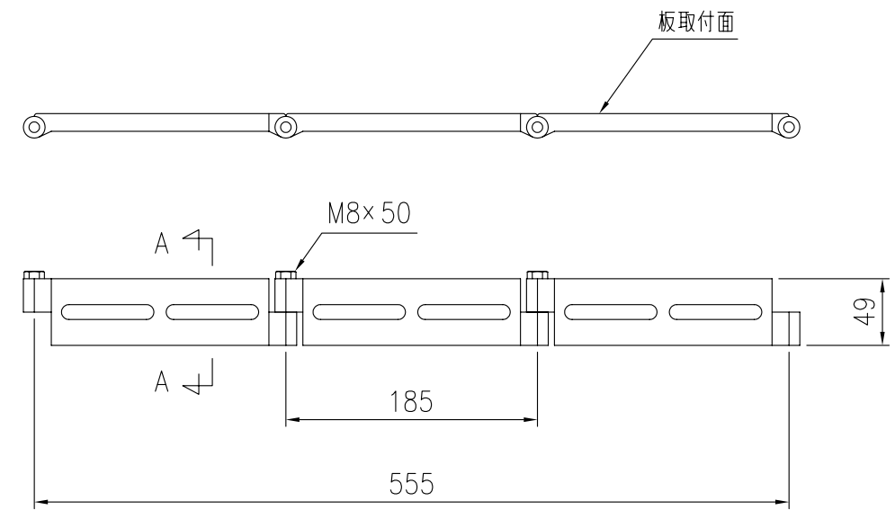
W取付金具詳細図 S=1/5
