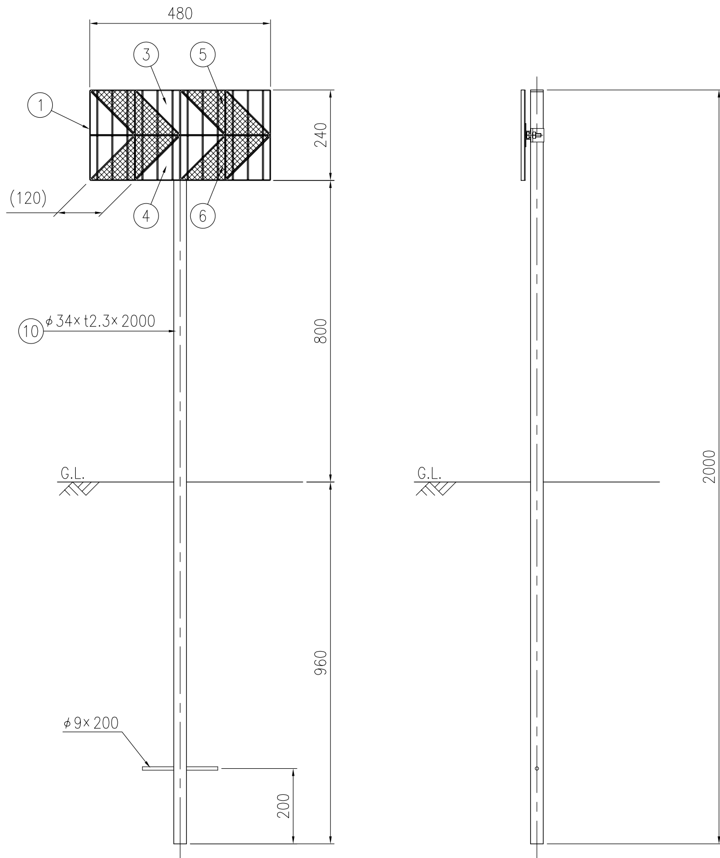
設置図 S=1/10
