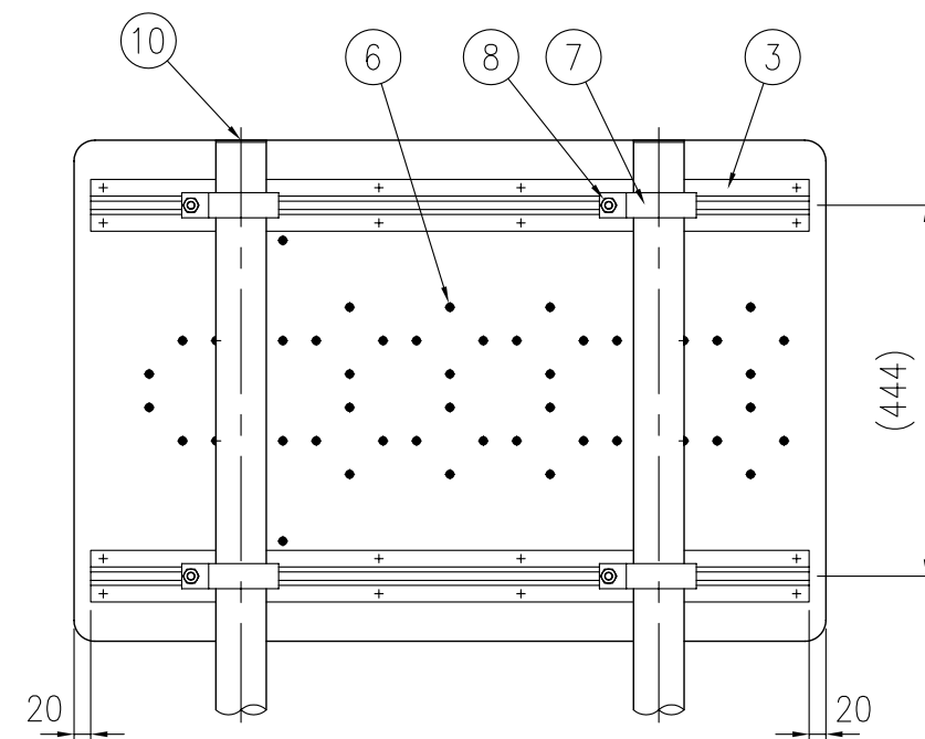
裏面図 S=1/10
