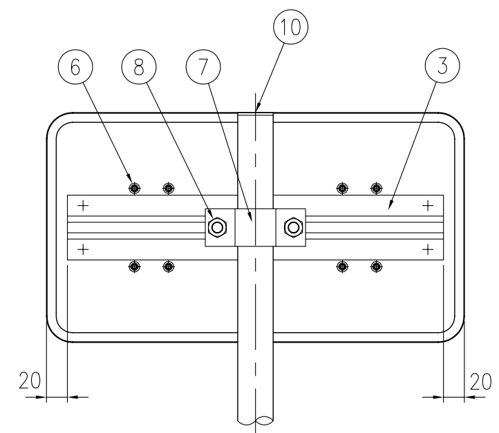
裏面図 S=1/5
