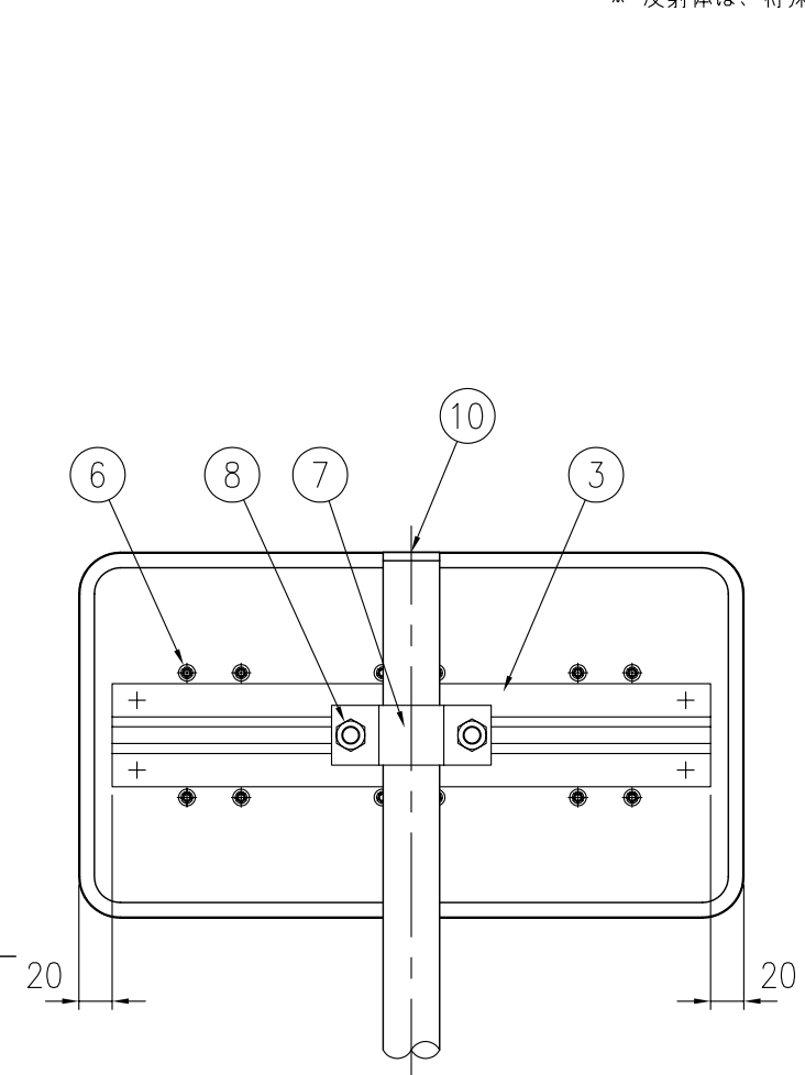
裏面図 S=1/5
