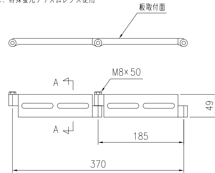
W取付金具詳細図 S=1/5
