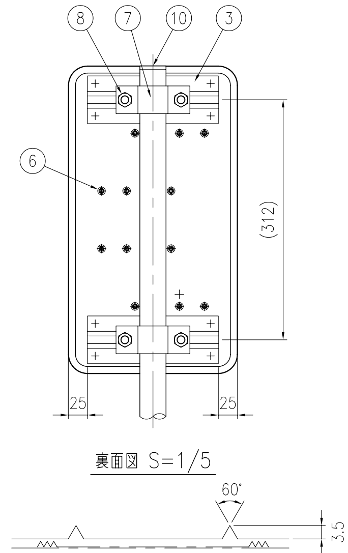
反射体突起部詳細図 S=1/1
