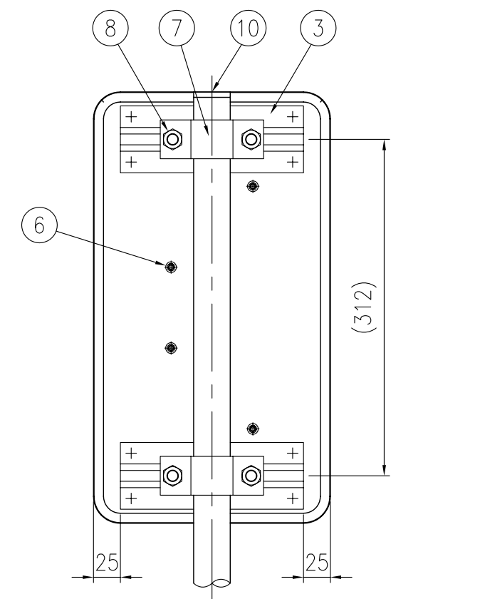
裏面図 S=1/5
