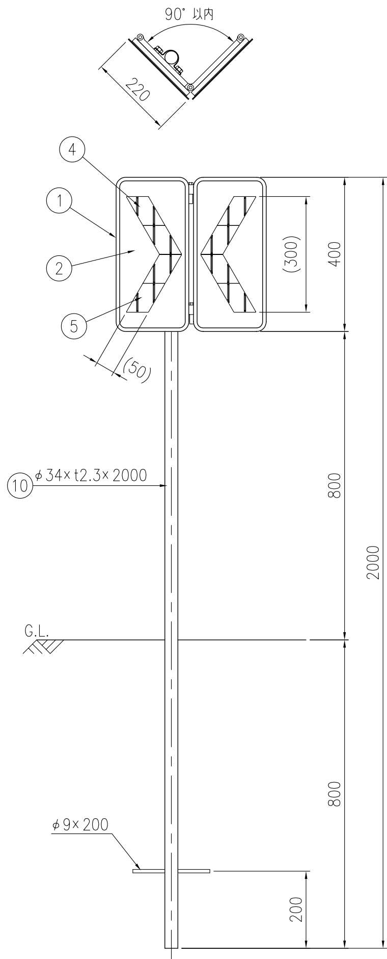
設置図 S=1/10
