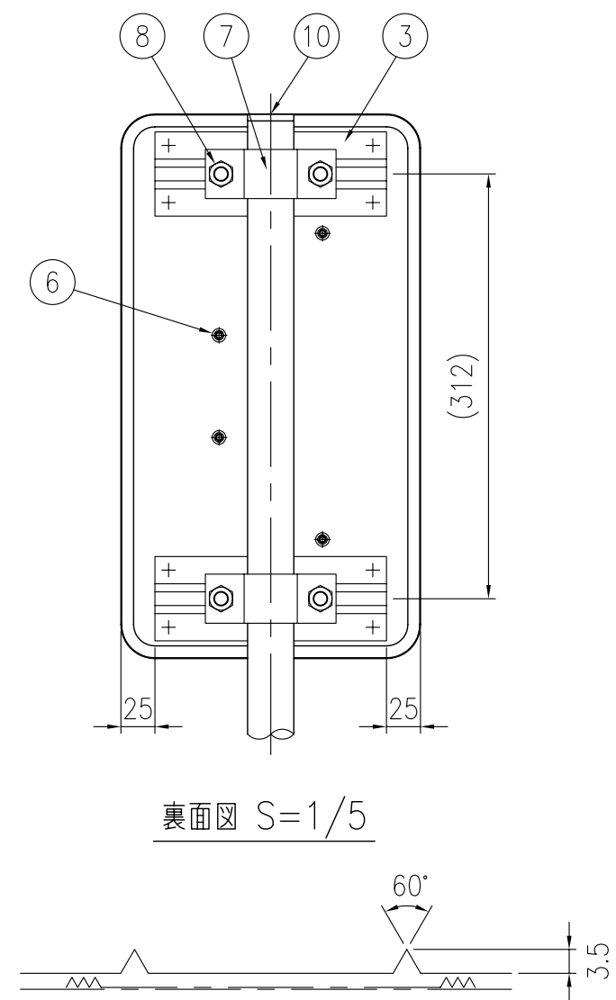
裏面図 S=1/5 反射体突起部詳細図 S=1/1
