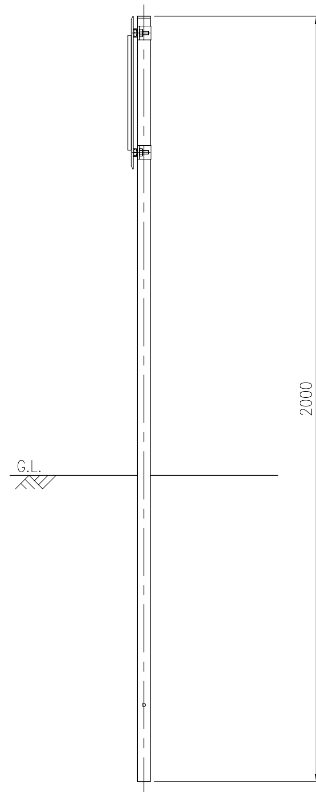
設置図 S=1/10
