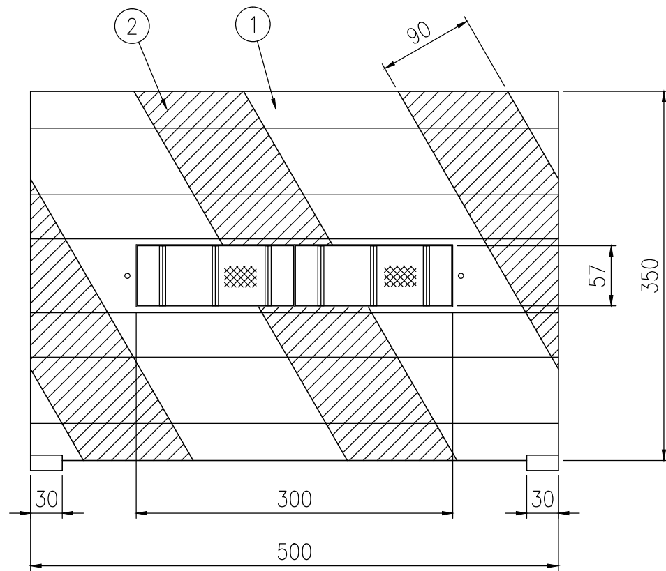
姿図 S=1/5
