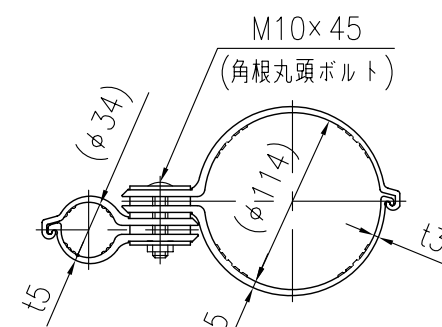
親子バンド詳細図 S=1/5
