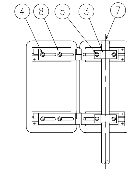
裏面図 S=1/10
