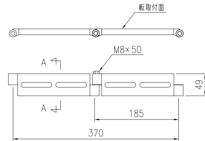
W取付金具詳細図 S=1/5
