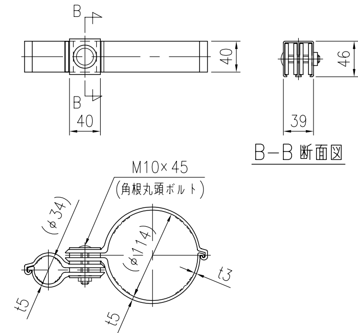
⑦親子バンド詳細図 S=1/5
