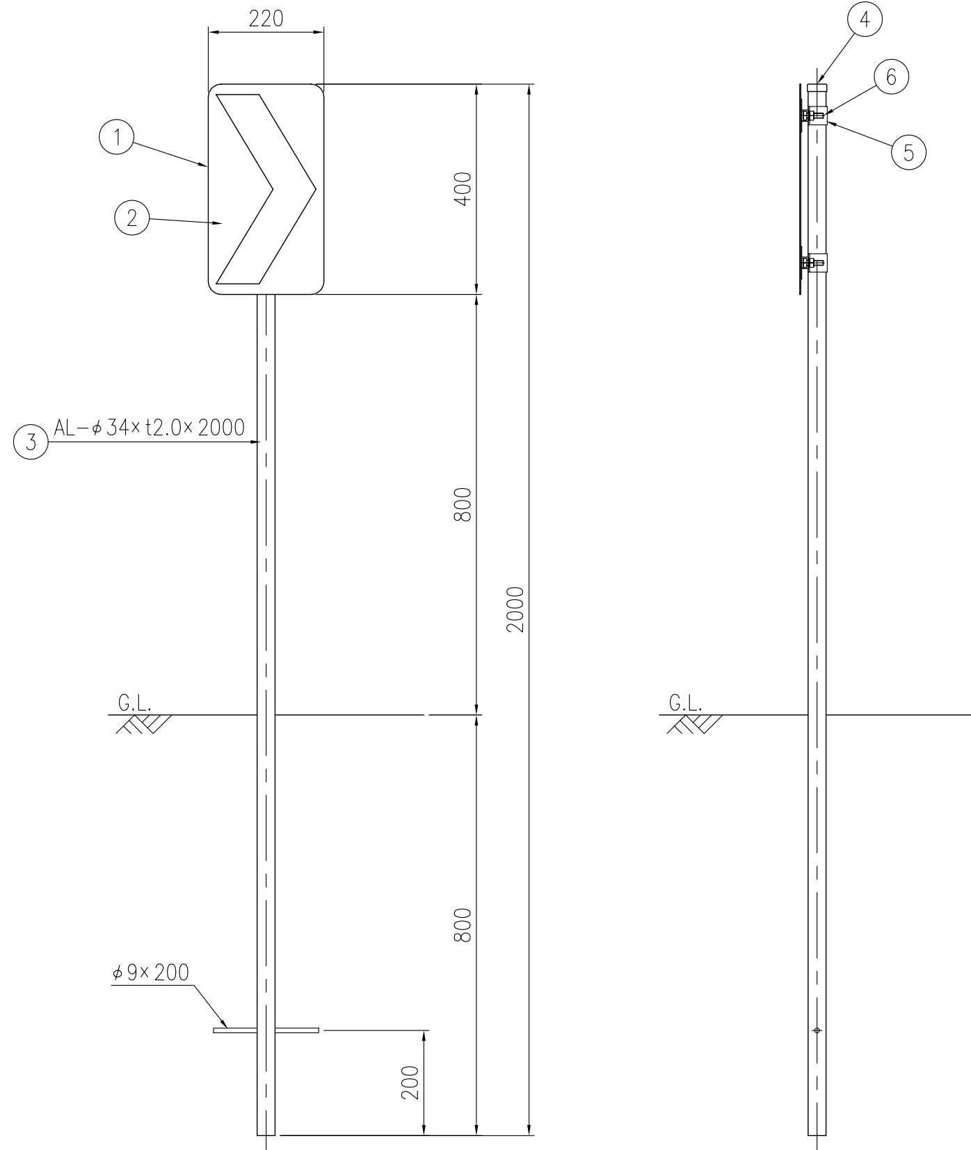
設置図 S=1/10
