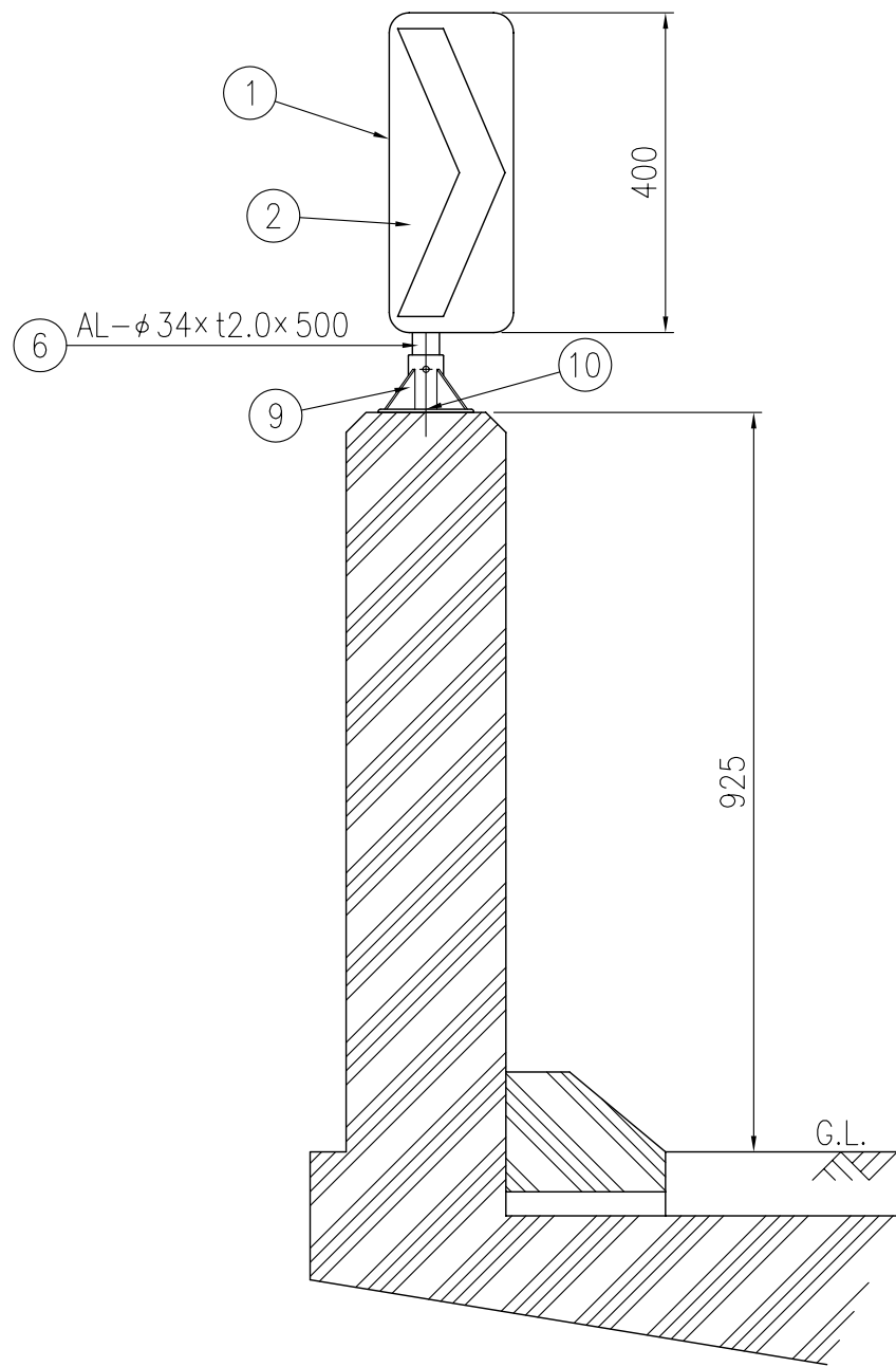
設置図 S=1/10
