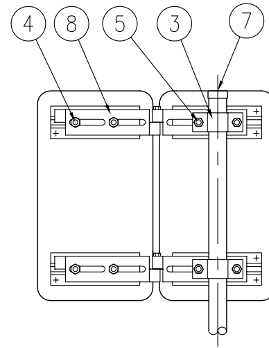
裏面図 S=1/10
