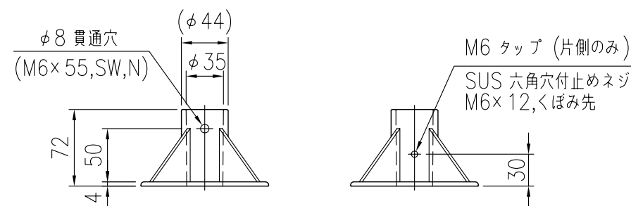
⑨ ベースプレート詳細図 S=1/5
