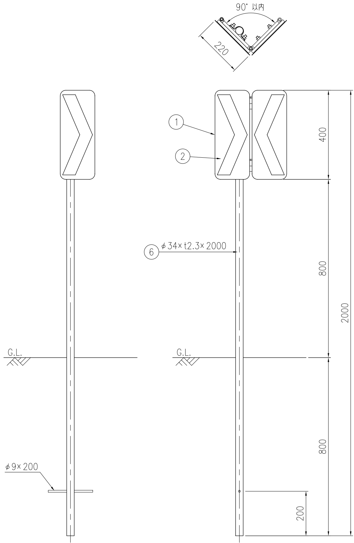
設置図 S=1/10
