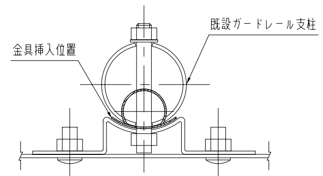
金具挿入位置 S=1/5
