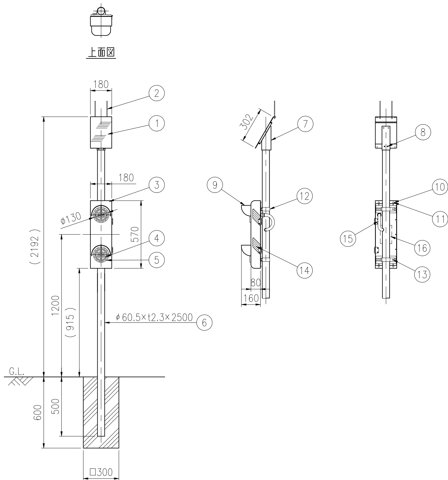
設置図 S=1/20
