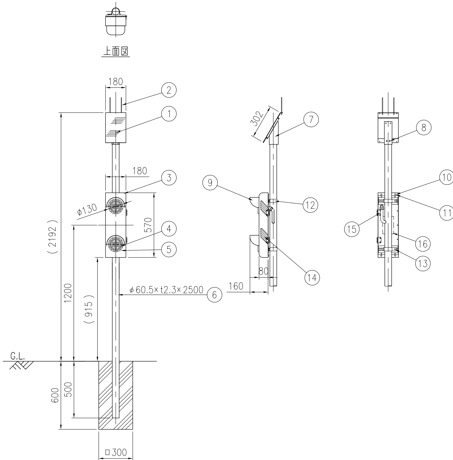
設置図 S=1/20
