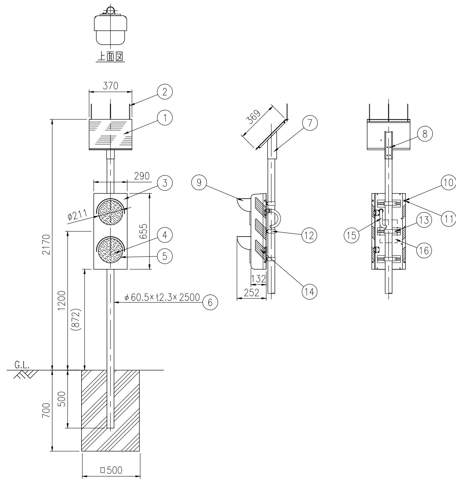
設置図 S=1/20
