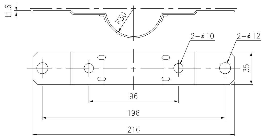
④ 取付金具詳細図 S=1/2
