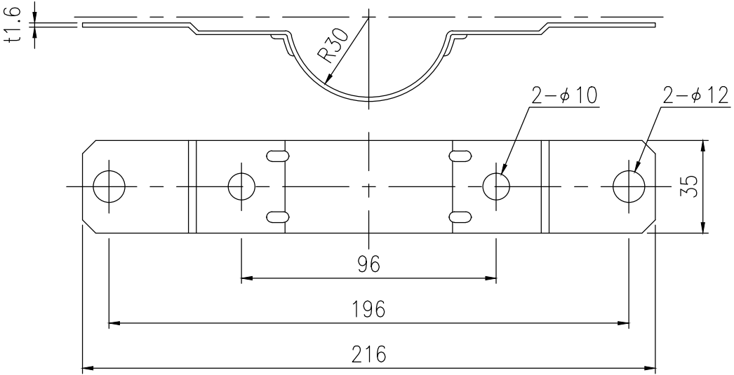
④ 取付金具詳細図 S=1/2
