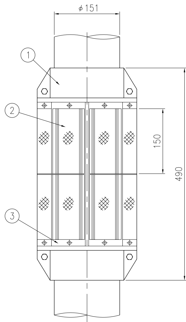
設置図 S=1/5
