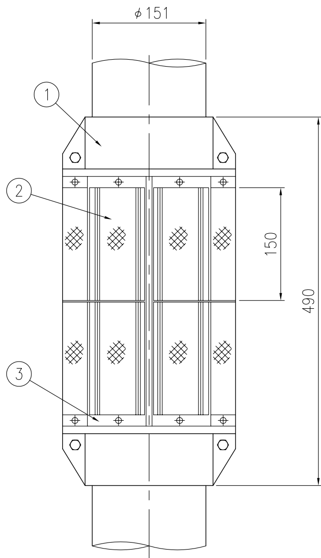
設置図 S=1/5
