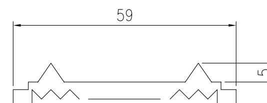
反射体突起部詳細図 S=1/1
