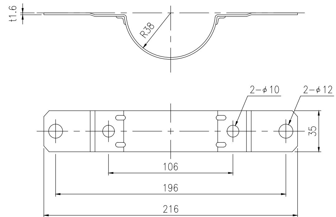
④ 取付金具詳細図 S=1/2
