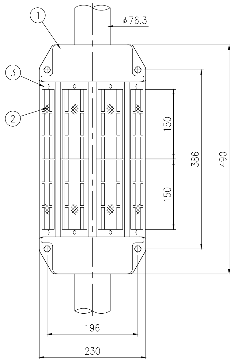
設置図 S=1/5
