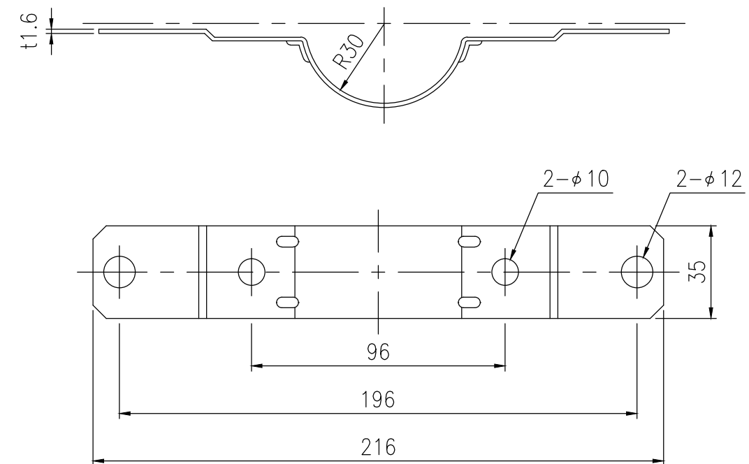
④ 取付金具詳細図 S=1/2
