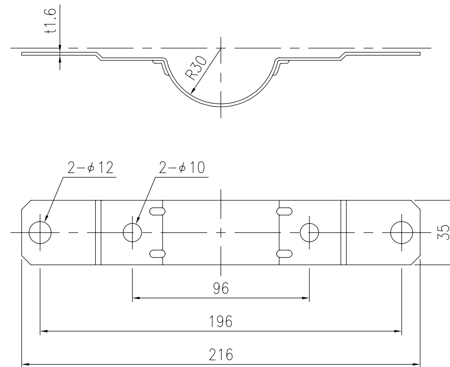
④ 取付金具詳細図 S=1/2
