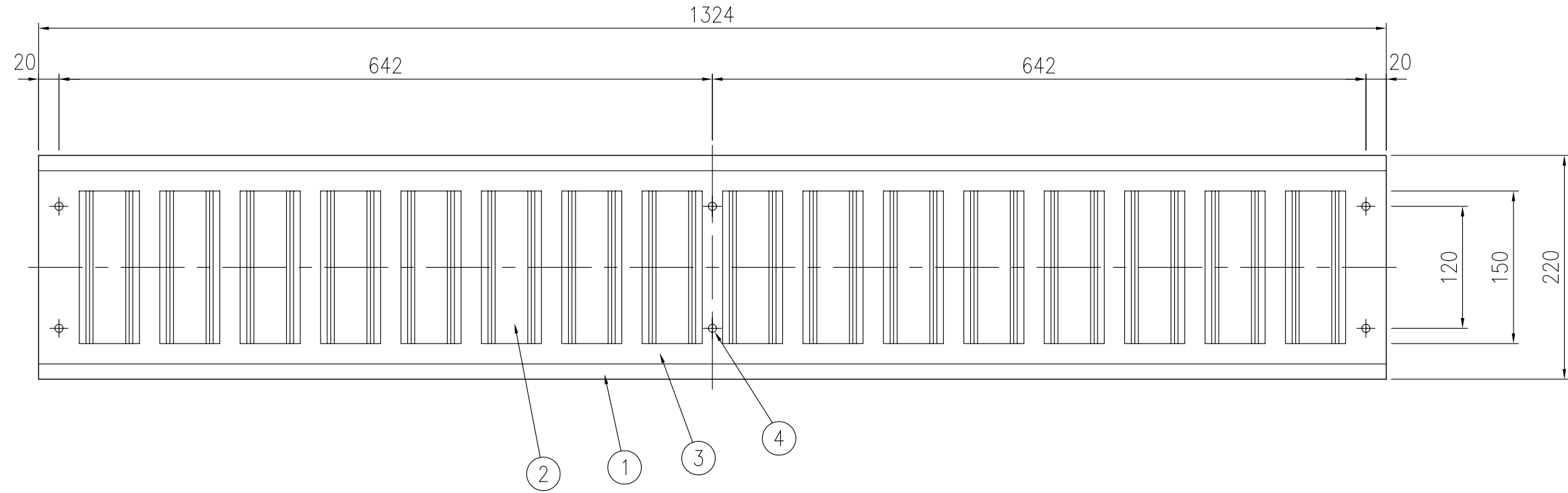
姿図 S=1/5
