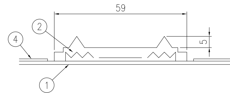
反射体突起部詳細図 S=1/1
