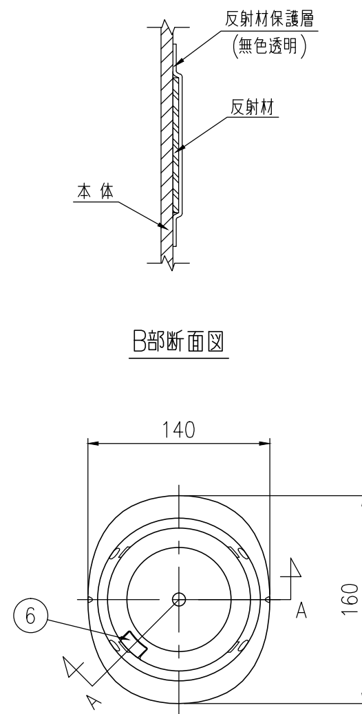
平面図 S=1/4
