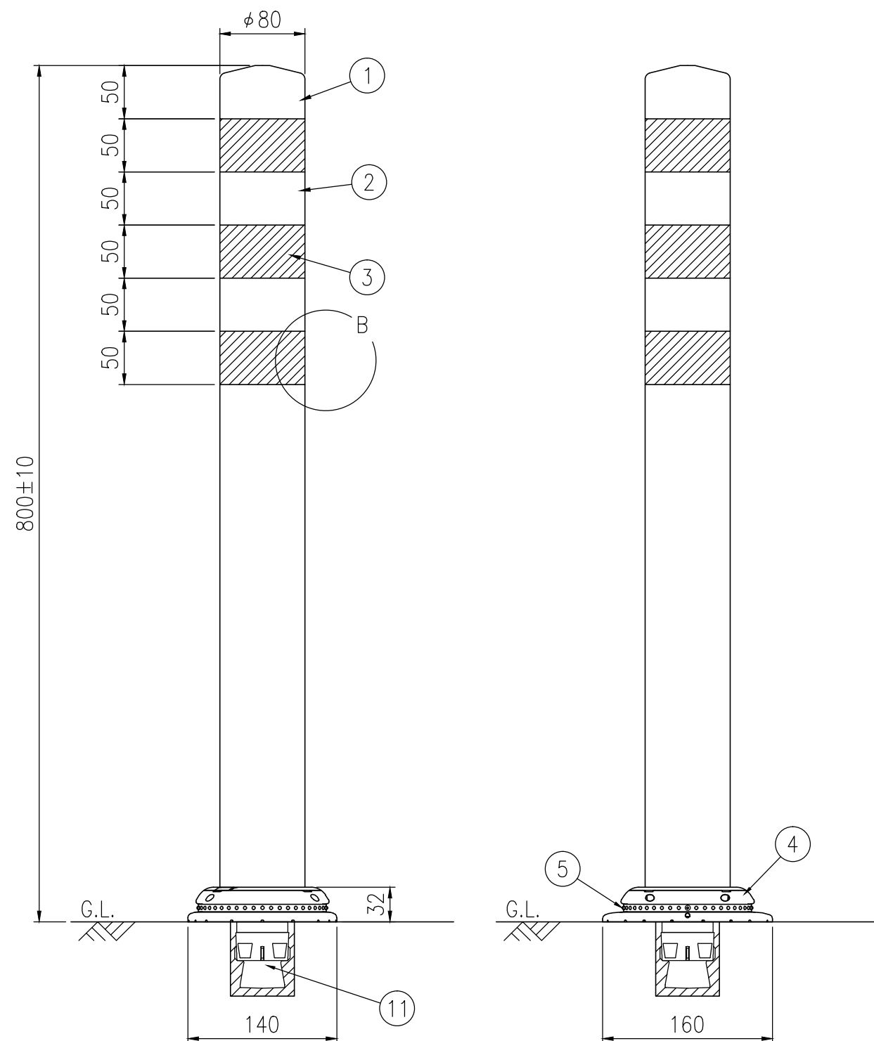
設置図 S=1/5
