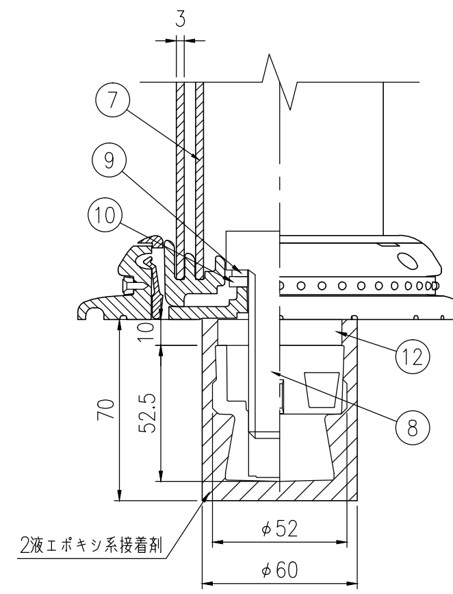
A-A半断面図 S=1/2
