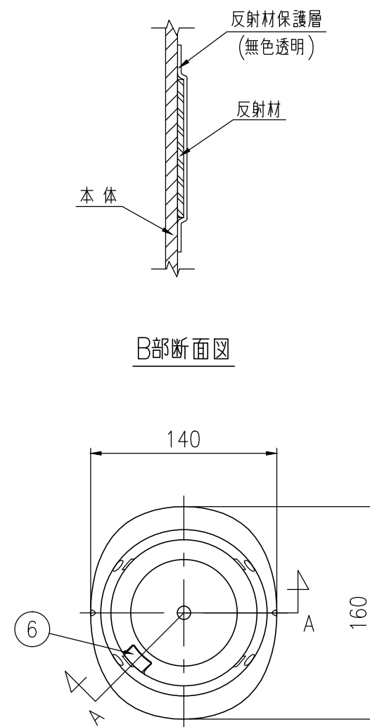
平面図 S=1/4
