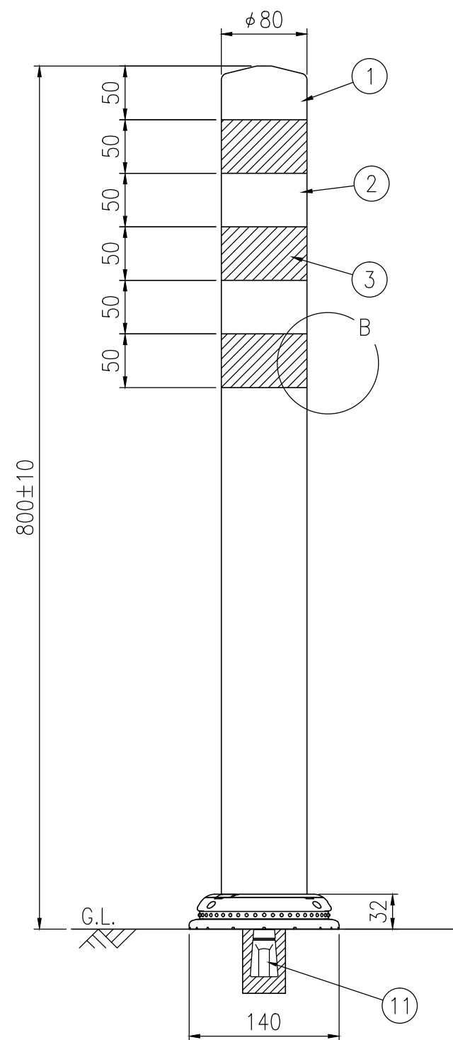
設置図 S=1/5
