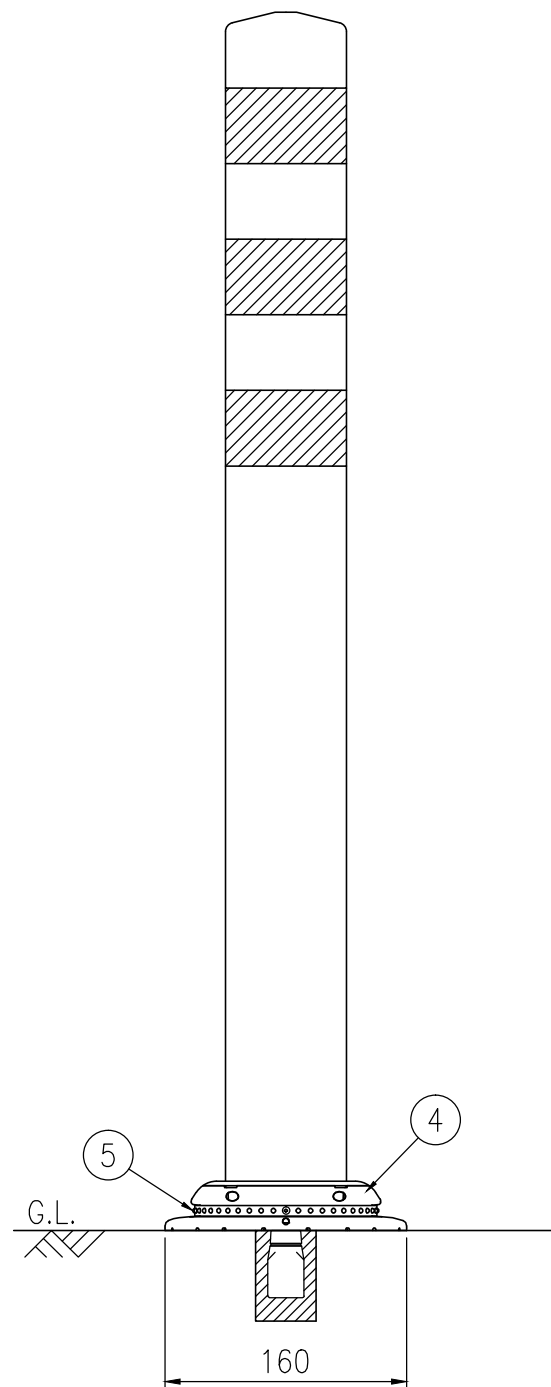
設置図 S=1/5
