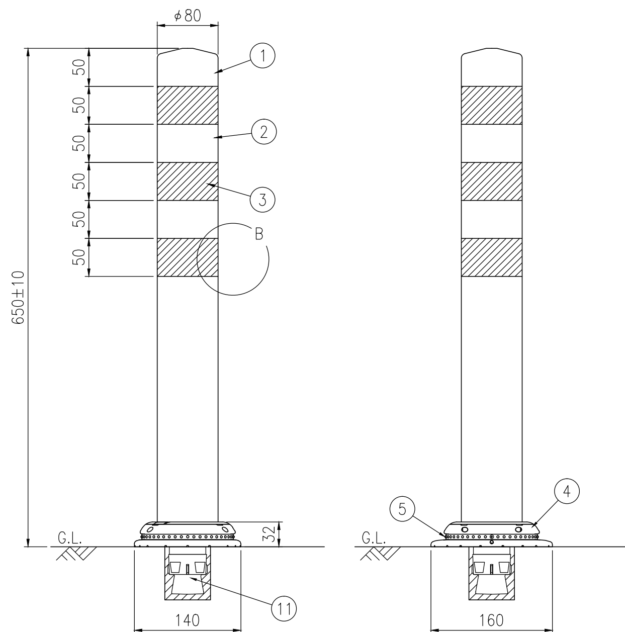
設置図 S=1/5
